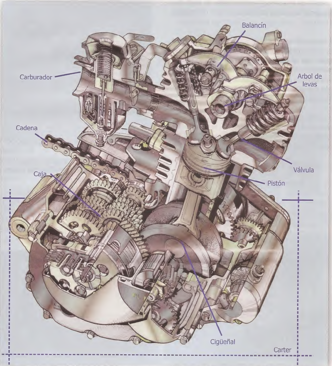
Corte de motor de cuatro tiempos
